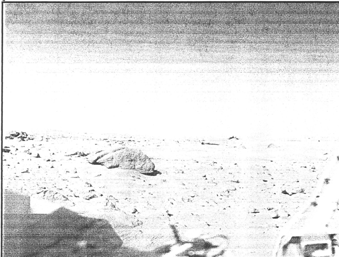
En vy av Mars taget av Viking 1 1979.
